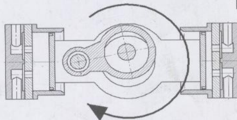
Esempio schematico di scorrimento assiale del pistone COMPACT-AIR 280 Example: COMPACT AIR 280 piston axial sliding
