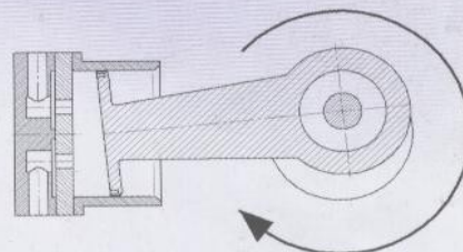
Esempio schematico di oscillazione dei pistoni conosciuti Example: well-known pistons oscillation
